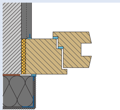
Fenster bündig mit dem Wandbildner
