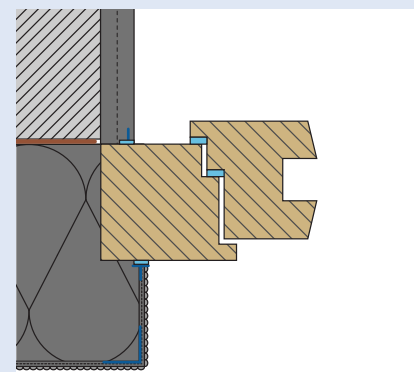
Fenster vor dem Wandbildner (im Dämmstoff) überputzbare Laibung erforderlich
